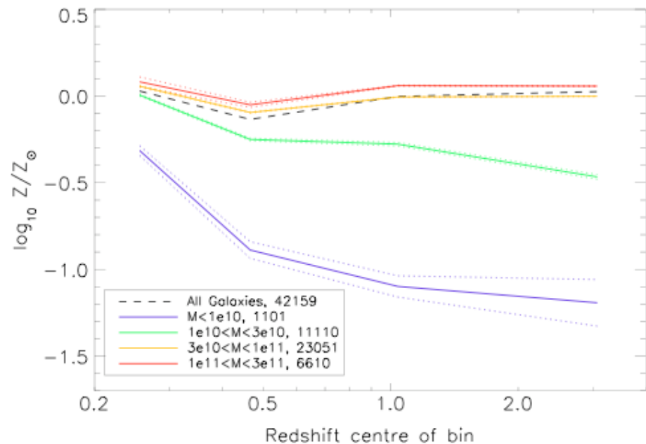
SDSS galaxies
